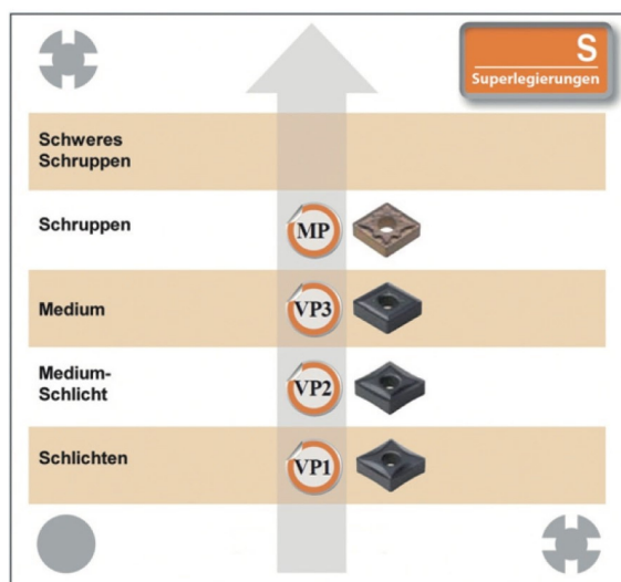
Spanbrecher für negative Wendepatten
