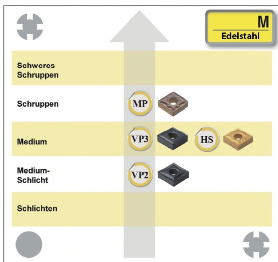
Spanbrecher für negative Wendepplatten
