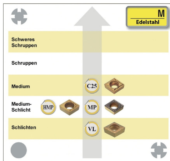
Spanbrecher für positive Wendepplatten
